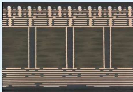
基板断面 (微細配線・積層技術)
