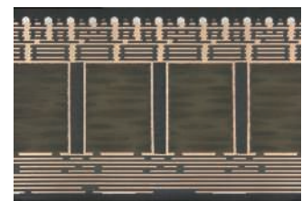
高多層化するデータセンター向け ICパッケージ基板(断面図)
